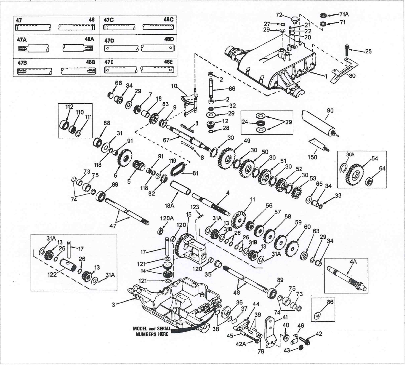
p801 801-801-038B / Transaxle
