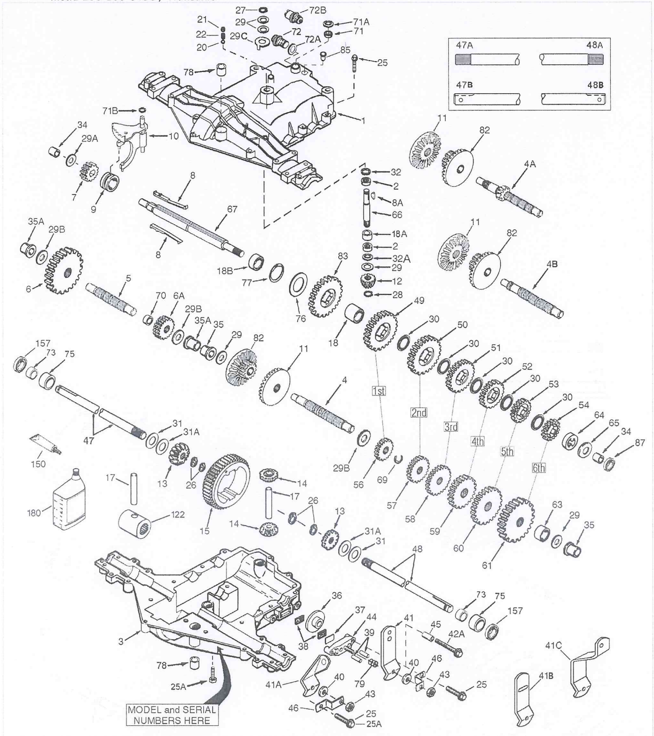
mst.2 206-206-545C / Transaxle
